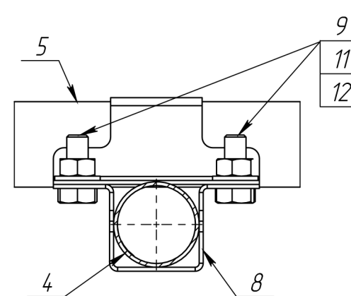
Б-Б (1 : 2)
