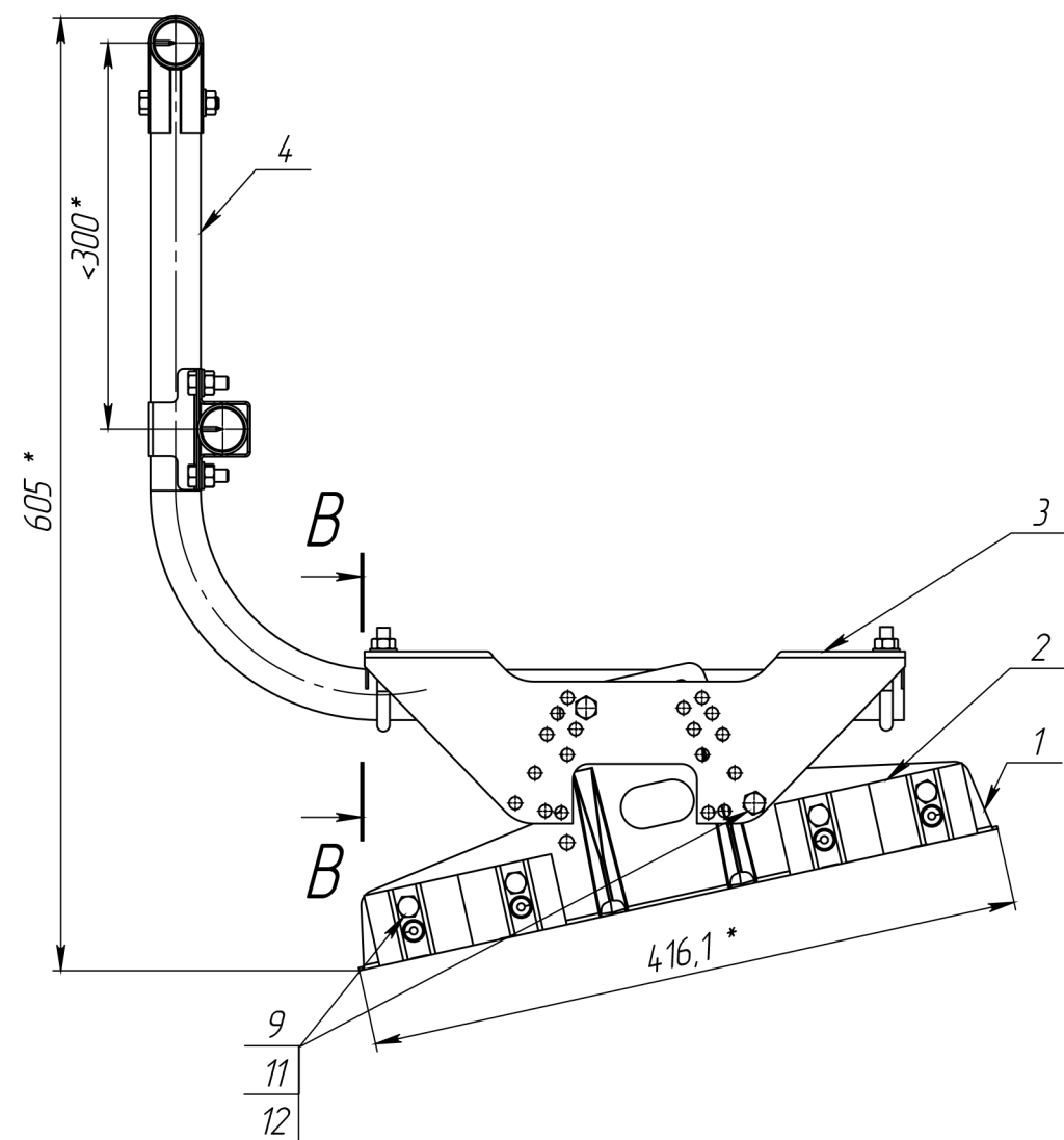
A (1 : 5)
