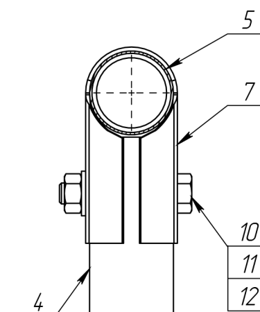
Г-Г (1 : 2)
